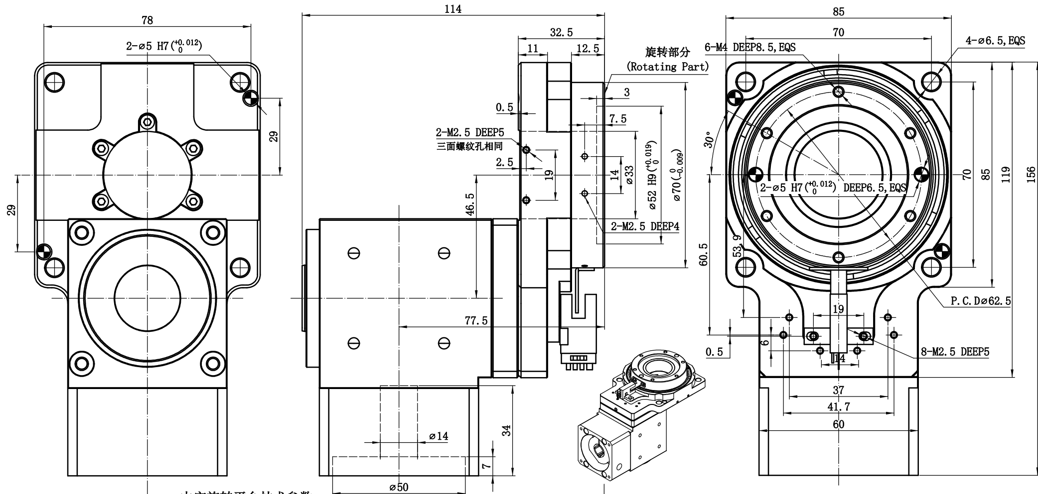
中空旋转平台技术参数 Technical Parameters of Planetary Reducer
